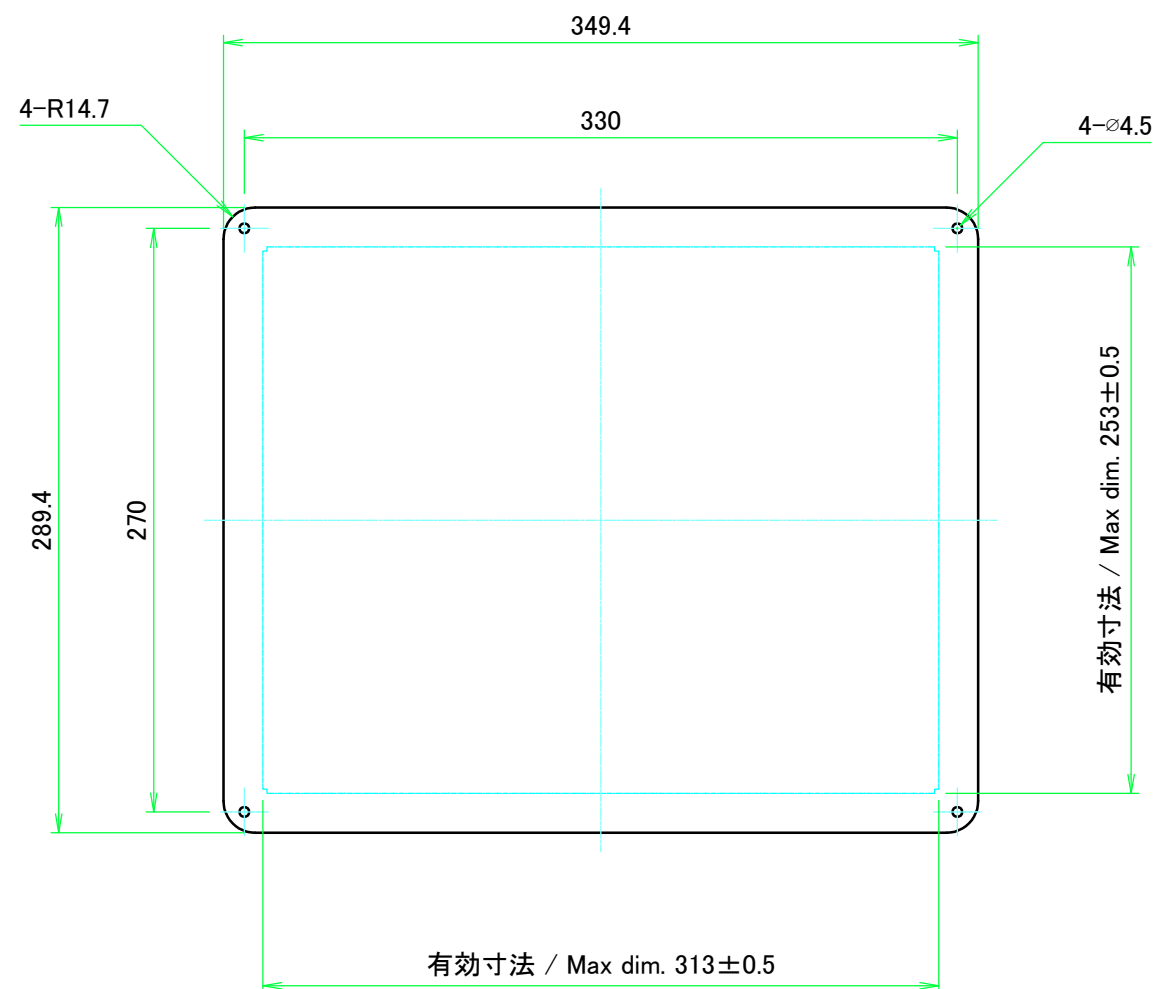
保護シート側 Surface protective film side
