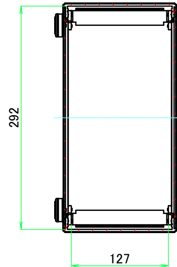
B-B ( 1 : 5 )
