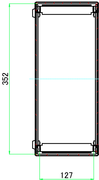
A-A ( 1 : 5.5 )
