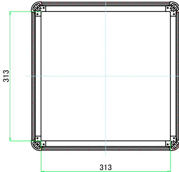
C-C ( 1 : 5.5 )
