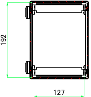
B-B ( 1 : 5.5 )
