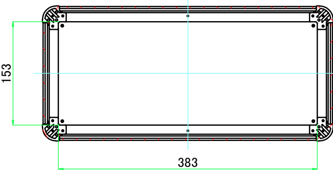
C-C ( 1 : 5.5 )
