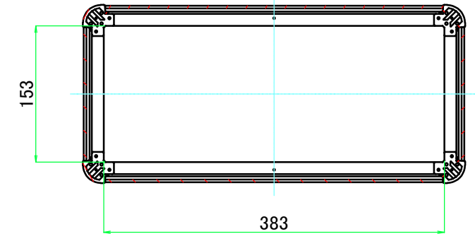
C-C ( 1 : 6 )
