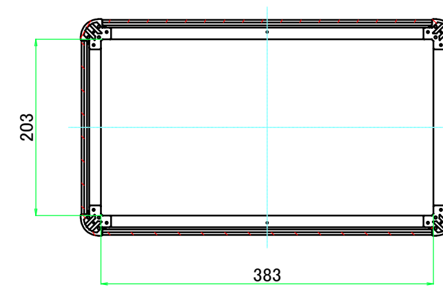
C-C ( 1 : 6 )
