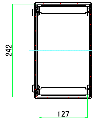
A-A ( 1 : 6 )
