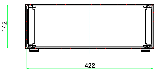
A-A (1:6.5)
