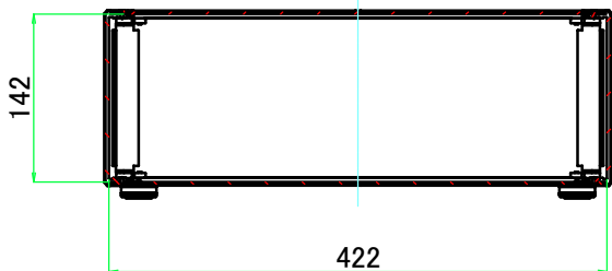
A-A ( 1 : 7 )
