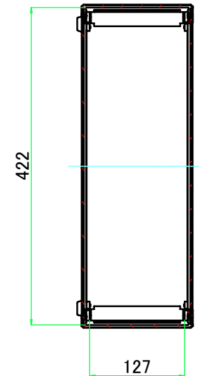
A-A ( 1 : 7 )
