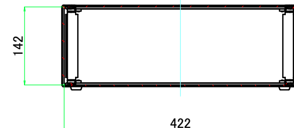
B-B ( 1 : 7 )
