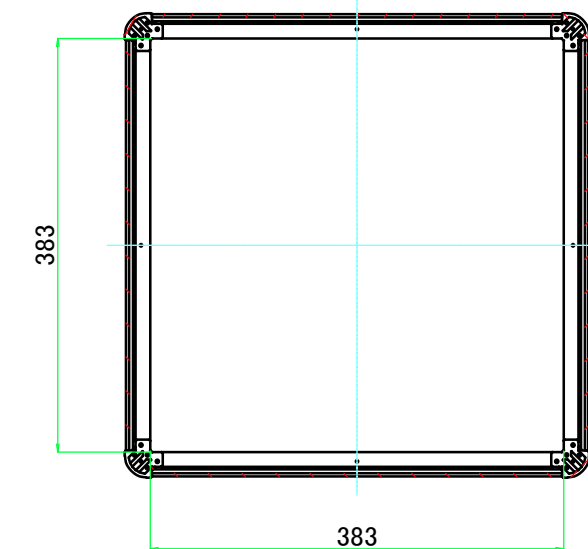
C-C ( 1 : 7 )
