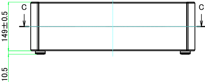
A-A ( 1 : 7 )
