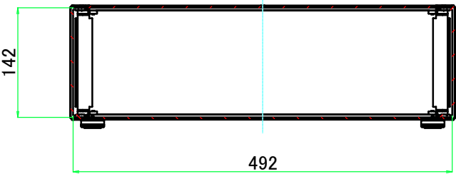
A-A ( 1 : 7 )
