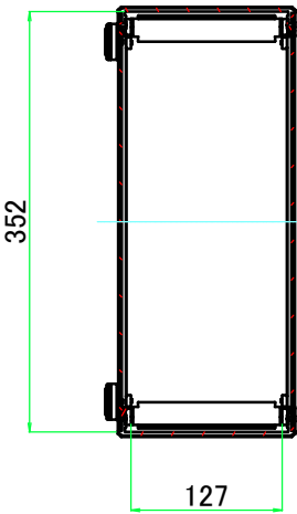
B-B ( 1 : 7 )
