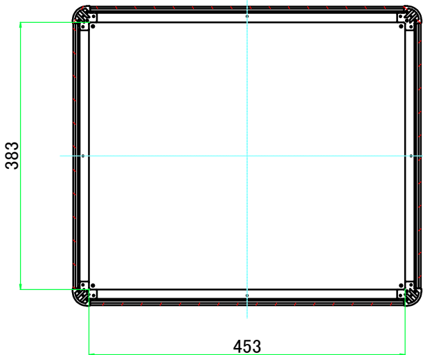
C-C ( 1 : 7.5 )
