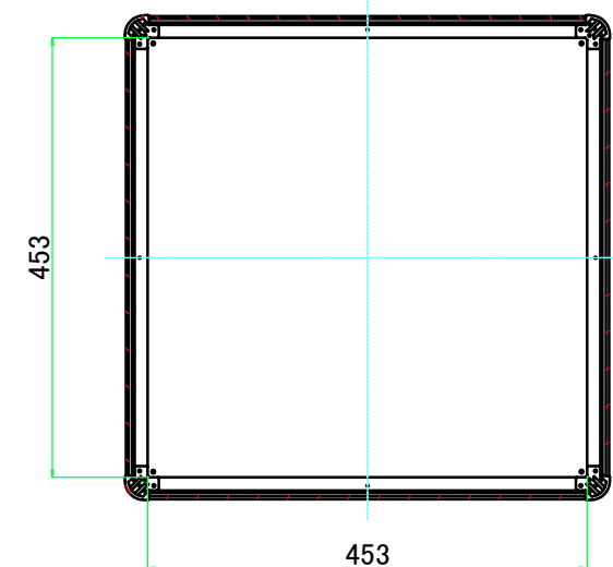
C-C ( 1 : 8.5 )
