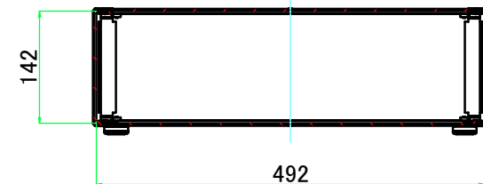
A-A ( 1 : 8.5 )
