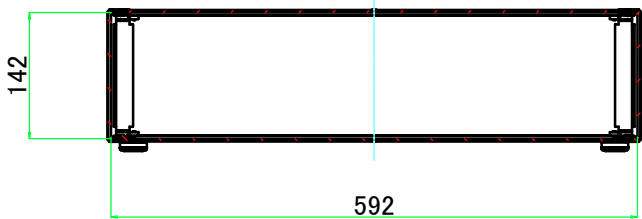
A-A ( 1 : 8.5 )
