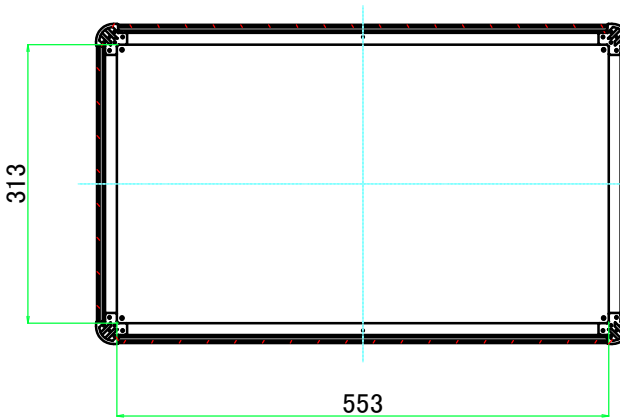
C-C ( 1 : 8.5 )
