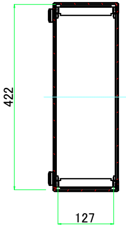
B-B ( 1 : 8.5 )
