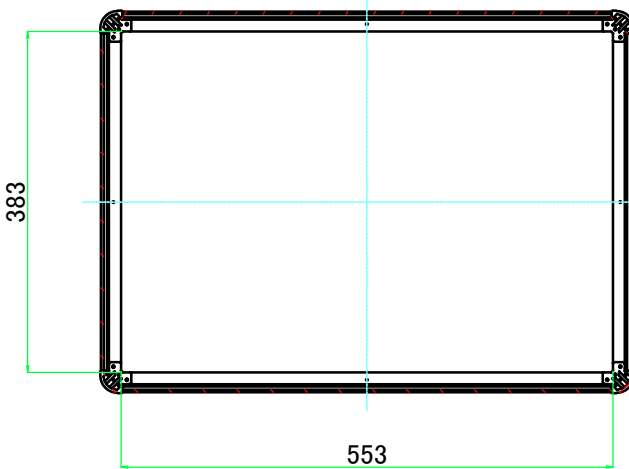
C-C ( 1 : 8.5 )
