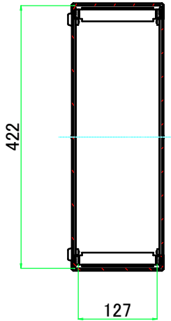
A-A ( 1 : 8.5 )
