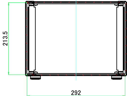
A-A ( 1 : 5.5 )
