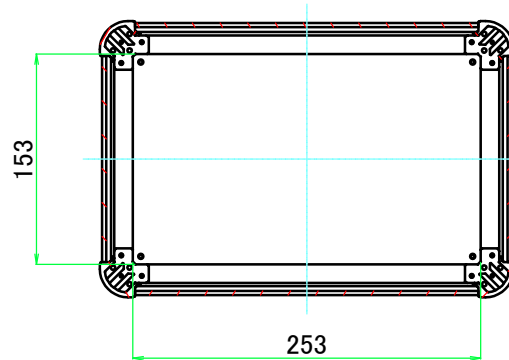
C-C ( 1 : 5.5 )
