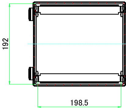
B-B ( 1 : 5.5 )
