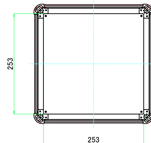
C-C ( 1 : 5.5 )
