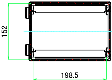
B-B ( 1 : 6 )
