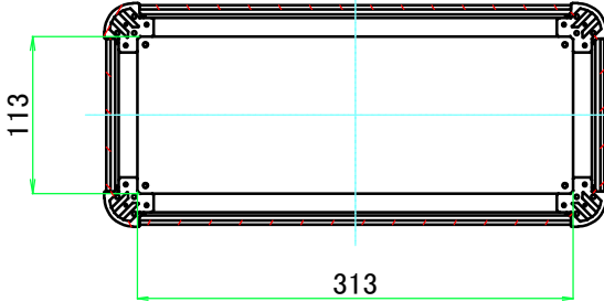
C-C ( 1 : 6 )
