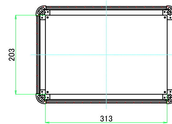
C-C ( 1 : 6 )
