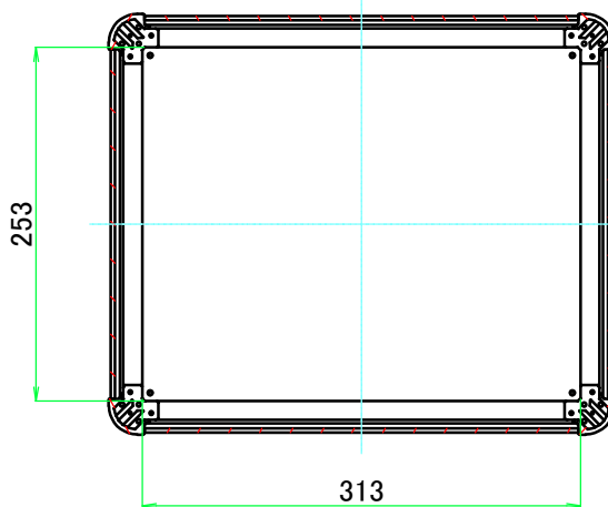
C-C ( 1 : 6 )
