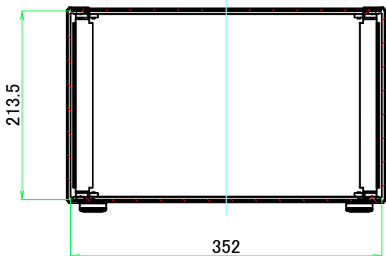
A-A ( 1 : 6 )
