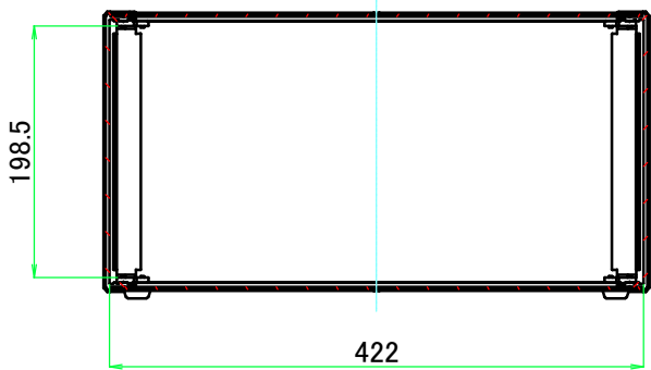
B-B ( 1 : 6.5 )
