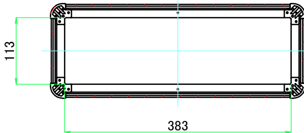
C-C ( 1 : 6.5 )
