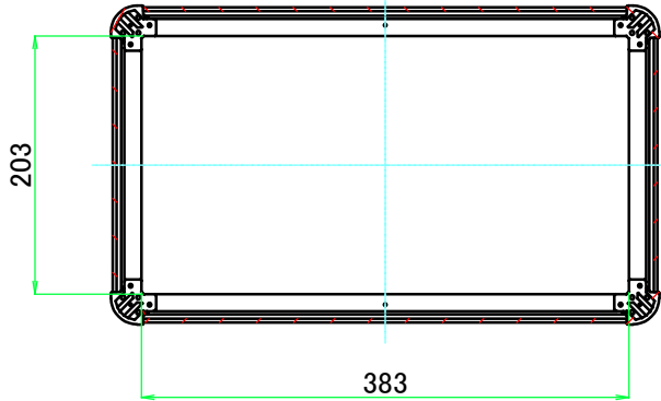
C-C ( 1 : 6.5 )
