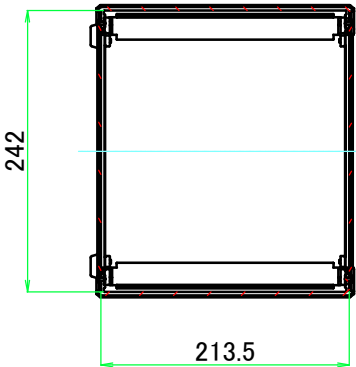
A-A ( 1 : 6.5 )
