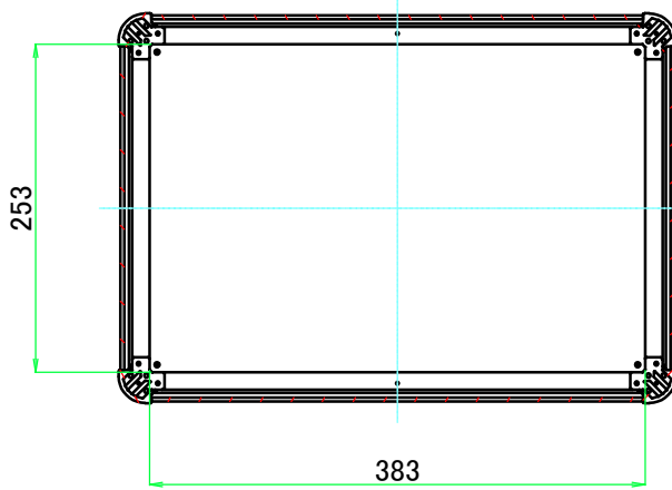
C-C ( 1 : 6.5 )
