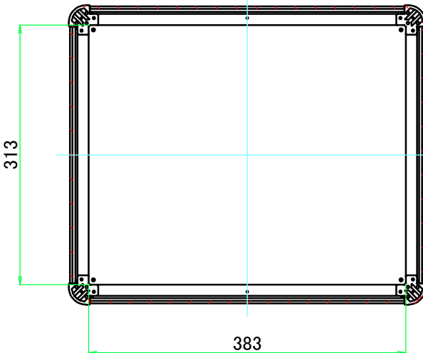
C-C ( 1 : 6.5 )
