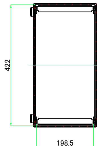
B-B ( 1 : 7.5 )
