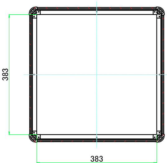
C-C ( 1 : 7.5 )
