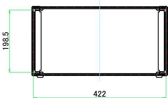
B-B ( 1 : 7.5 )
