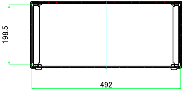
B-B ( 1 : 7.5 )
