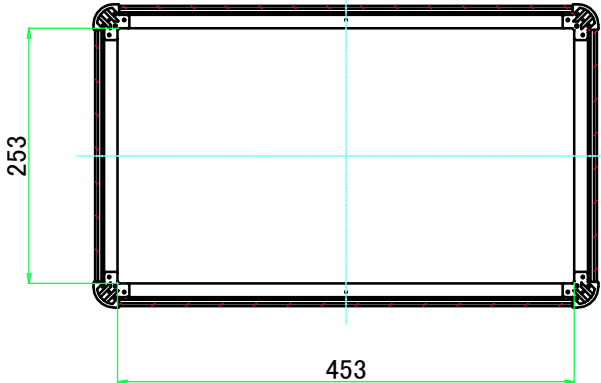
C-C ( 1 : 7.5 )
