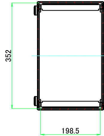
B-B ( 1 : 7.5 )
