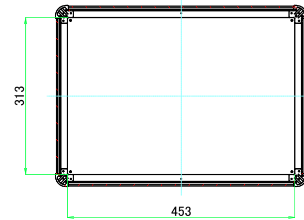
C-C ( 1 : 7.5 )
