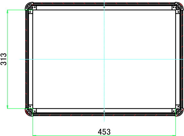
C-C ( 1 : 7.5 )
