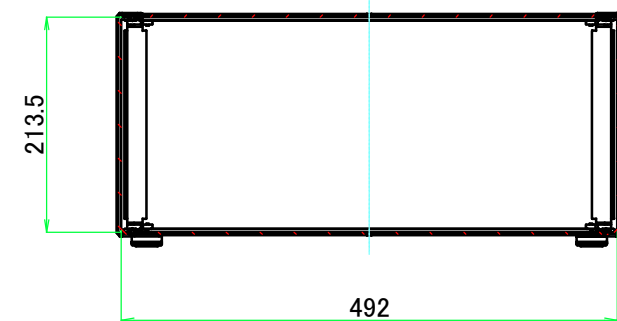
A-A ( 1 : 7.5 )
