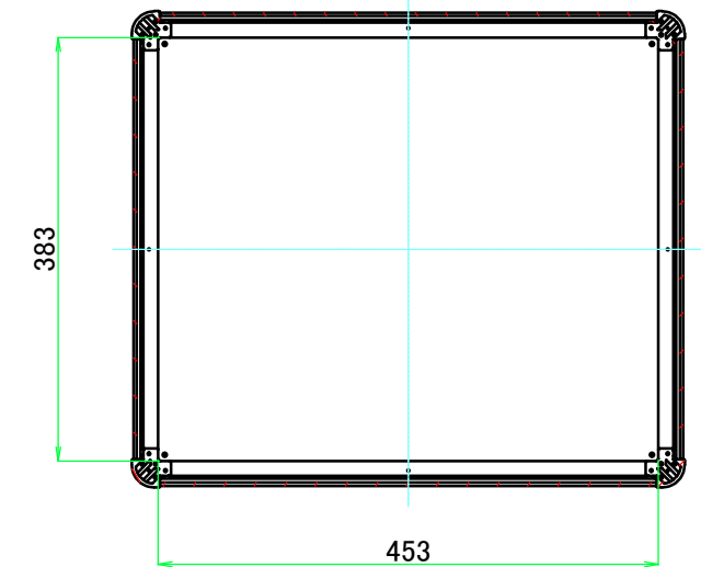
C-C ( 1 : 7.5 )
