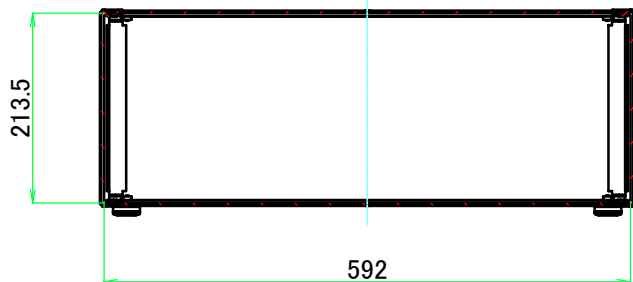
A-A ( 1 : 8.5 )
