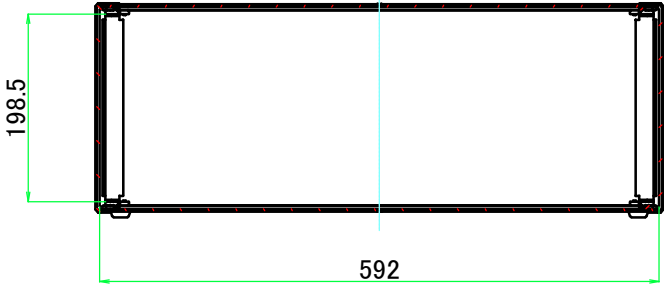
B-B ( 1 : 8 )
