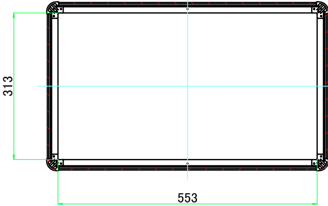
C-C ( 1 : 8 )
