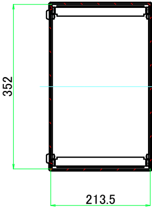
A-A ( 1 : 8 )
