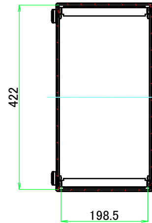
B-B ( 1 : 8.5 )
