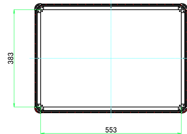
C-C ( 1 : 8.5 )
