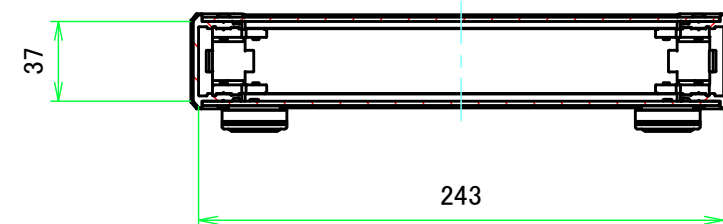
B-B (1 : 3.5)
