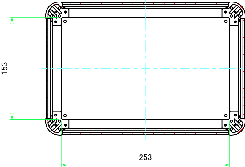
C-C (1:3.5)
