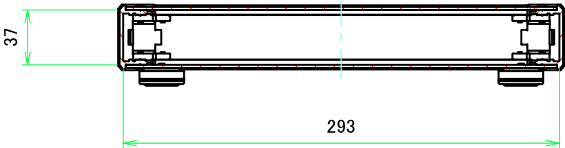
B-B (1:3.5)
