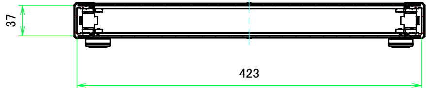
B-B ( 1 : 4.5 )
