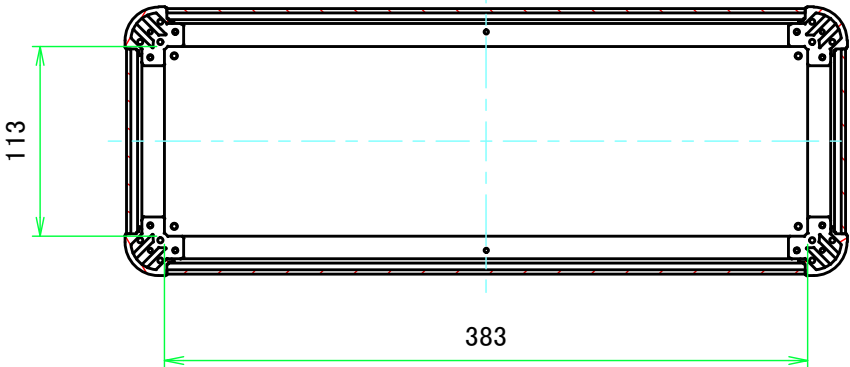
C-C ( 1 : 4.5 )
