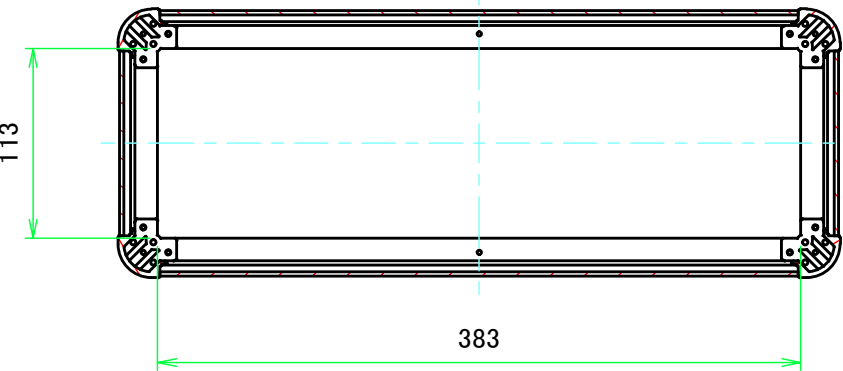
C-C ( 1 : 4.5 )
