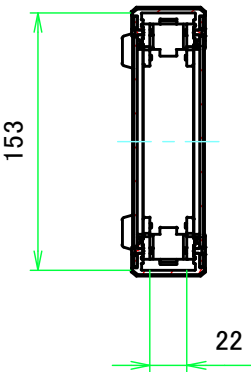
A-A ( 1 : 4.5 )
