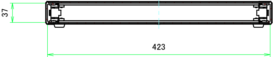
B-B ( 1 : 4.5 )
