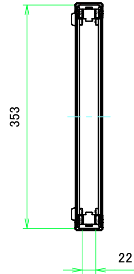
A-A (1:6)
