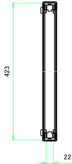
A-A (1:6)
