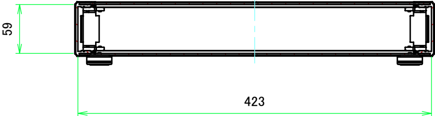
B-B ( 1 : 4.5 )
