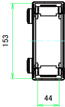
A-A ( 1 : 4.5 )
