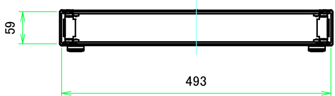
B-B ( 1:7 )
