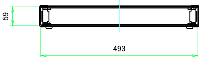
B-B ( 1:7 )
