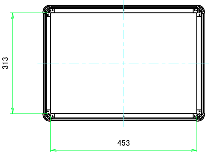
C-C ( 1:7 )
