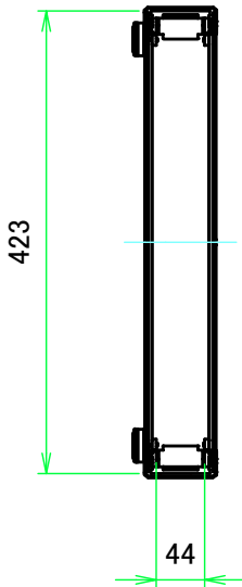
A-A ( 1:7.5 )
