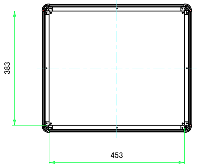
C-C ( 1:7.5 )
