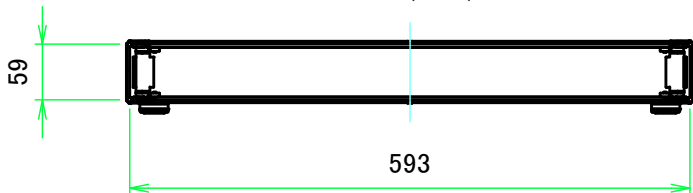
B-B ( 1:8 )
