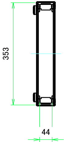
A-A ( 1:8 )
