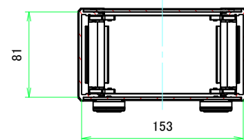
B-B (1:3.5)
