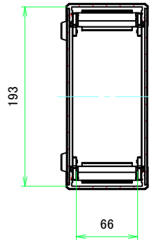
A-A (1:4)
