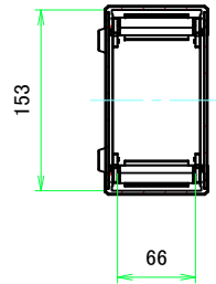
A-A (1:5)
