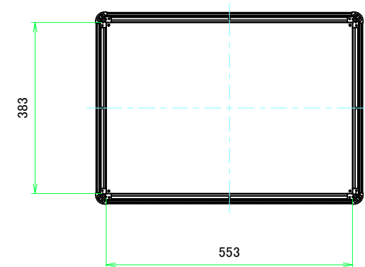
C-C (1 : 8.5)
