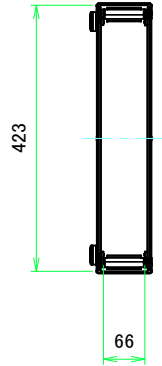
A-A (1 : 8.5)
