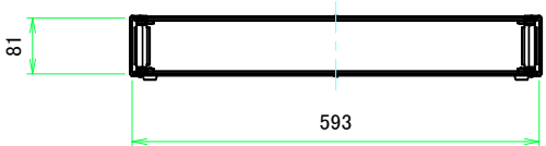
B-B ( 1 : 8.5 )
