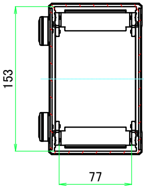
B-B ( 1 : 4 )
