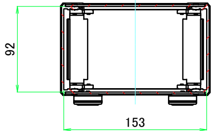
A-A ( 1 : 4 )
